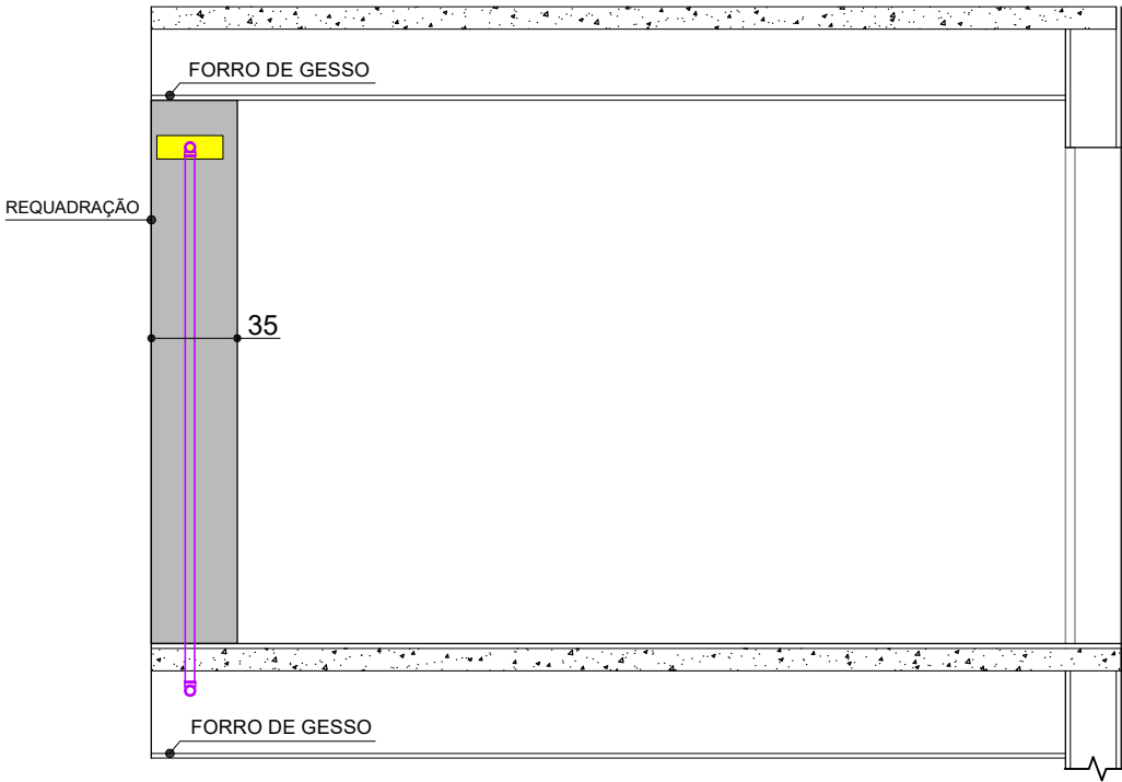
VISTA A
