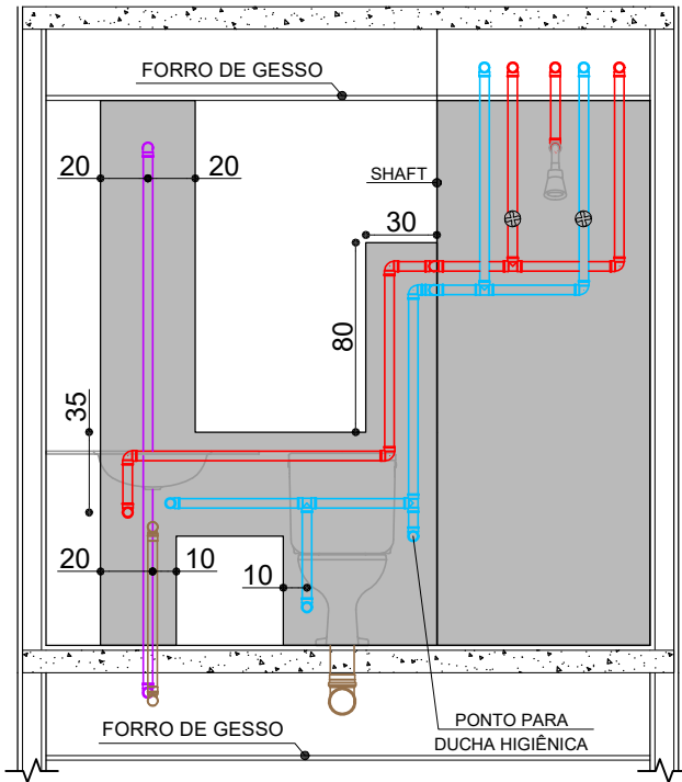
VISTA 1
