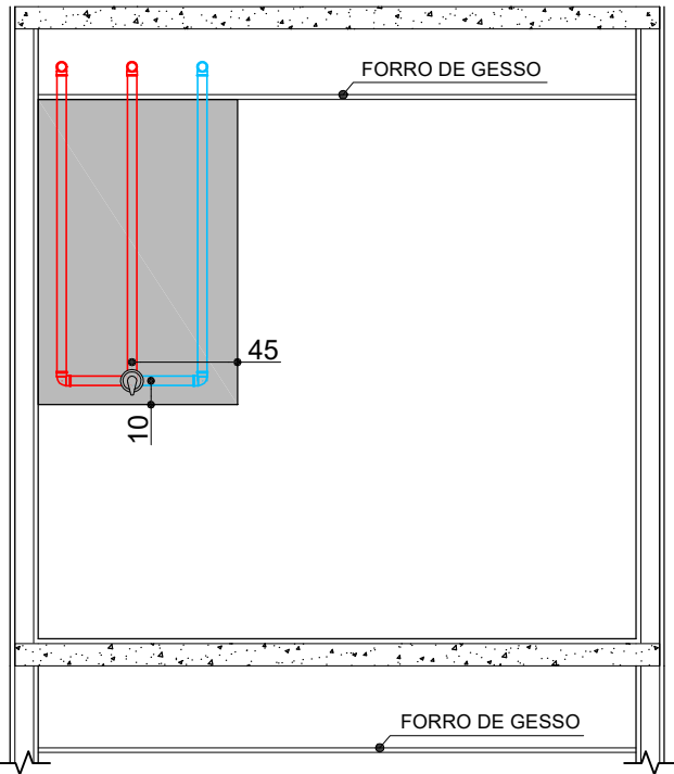
VISTA 2
