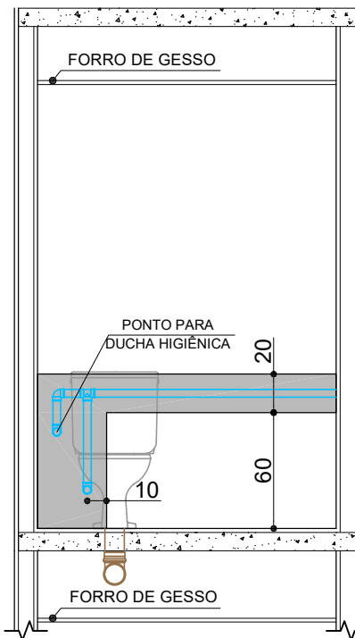
VISTA 1
