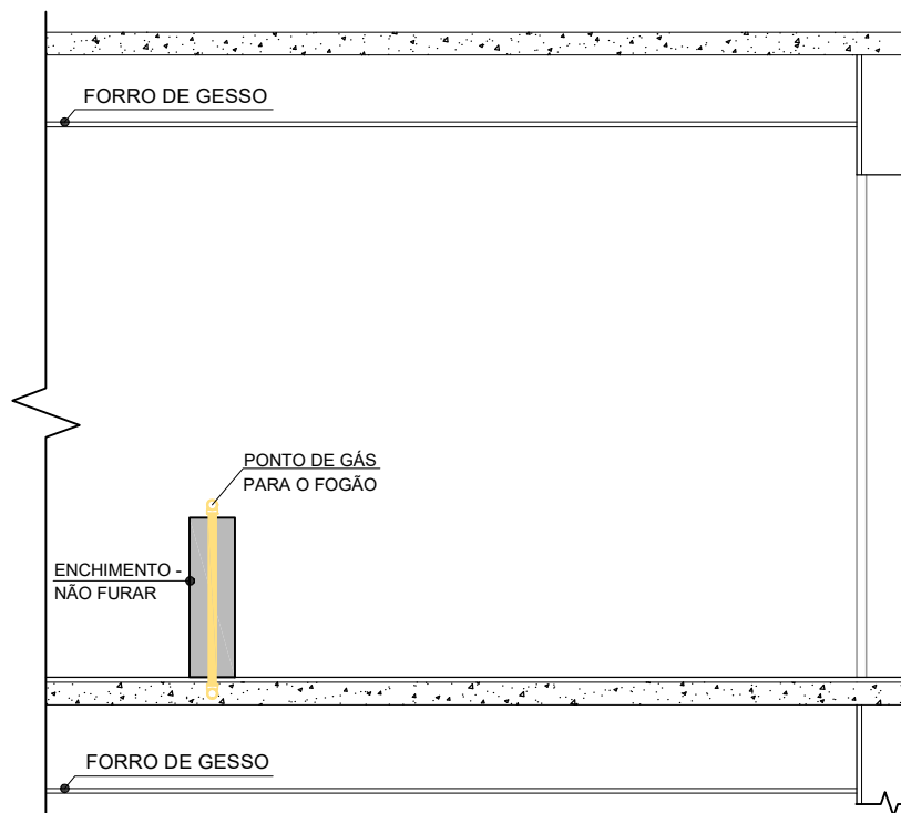
VISTA 1
