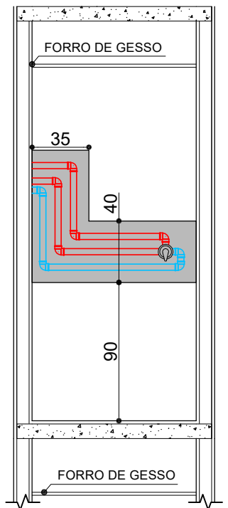
VISTA 3
