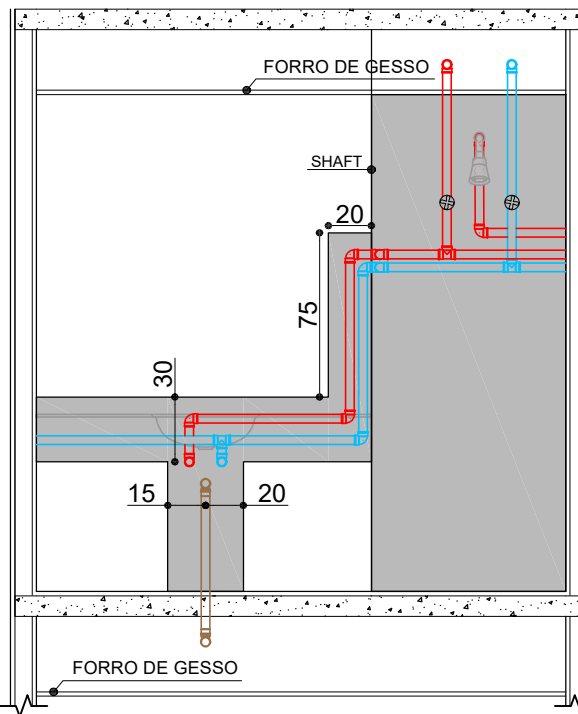
VISTA 2
