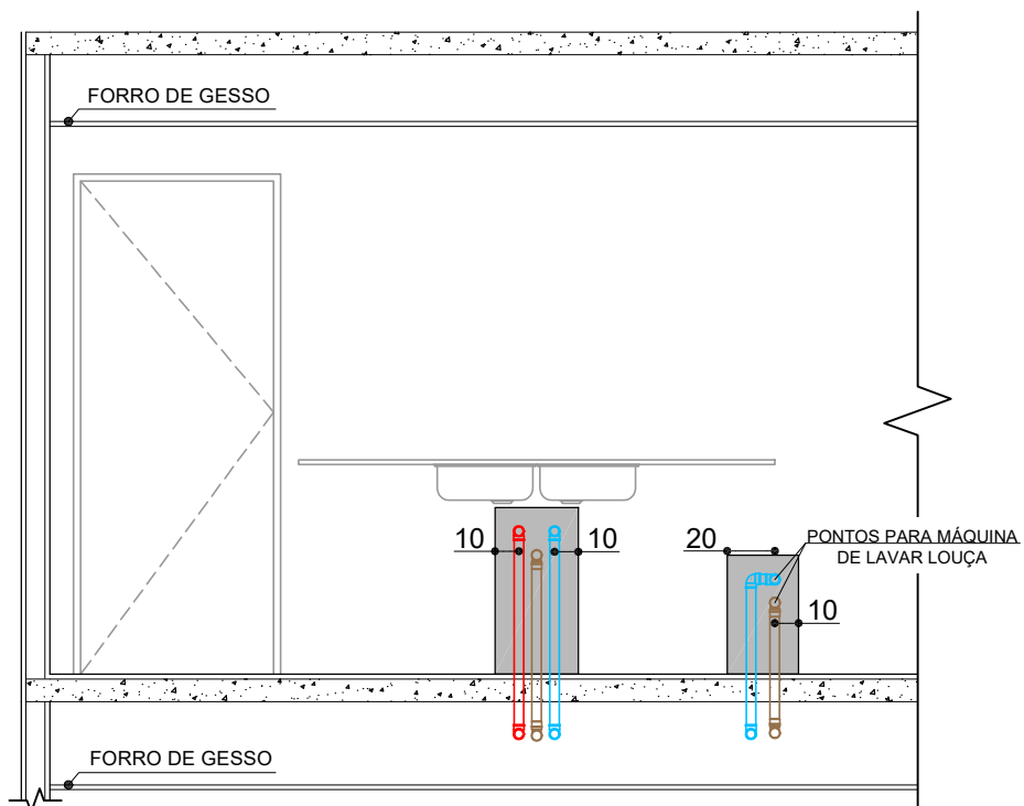
VISTA 1
